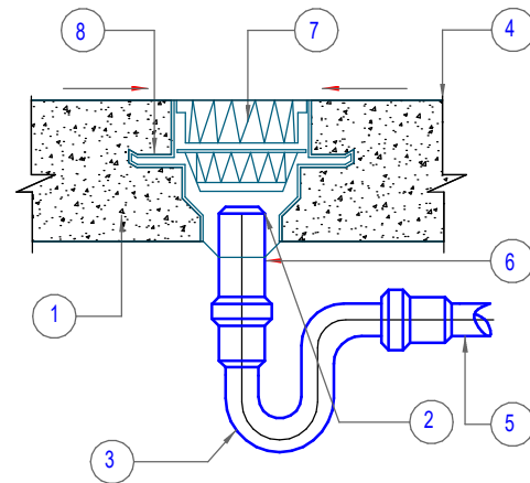
MẶT CẮT PHỄU THU NƯỚC
