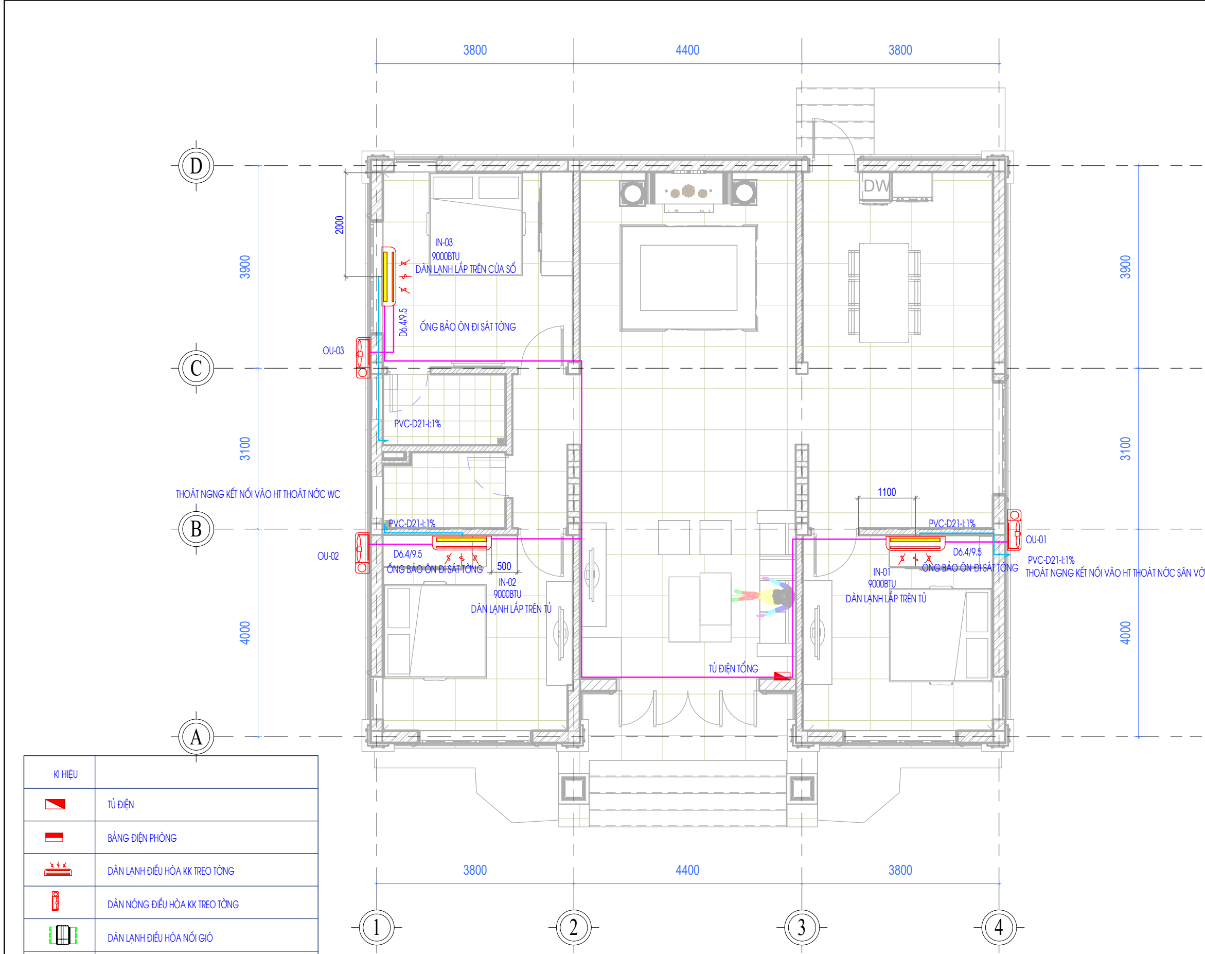
MẶT BẰNG CẤP ĐIỆN ĐIỀU HÒA TẦNG 1 TL: (1 : 75)
