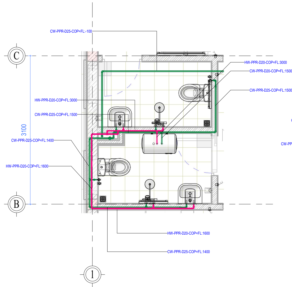
CHI TIẾT CẤP NƯỚC VỆ SINH TL: (1 : 40 )
