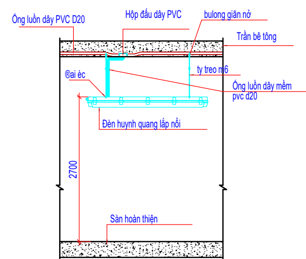
CHI TIẾT LẮP ĐẶT ĐÈN HUỖNH QUANG LẮP NỔI
