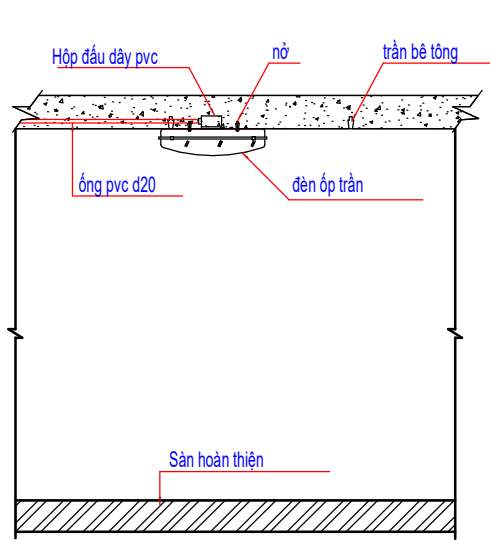
CHI TIẾT LẮP ĐẶT ĐÈN ỐP TRẦN
