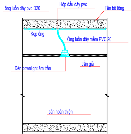
CHI TIẾT LẮP ĐẶT ĐÈN DOWNLIGHT ÂM TRẦN
