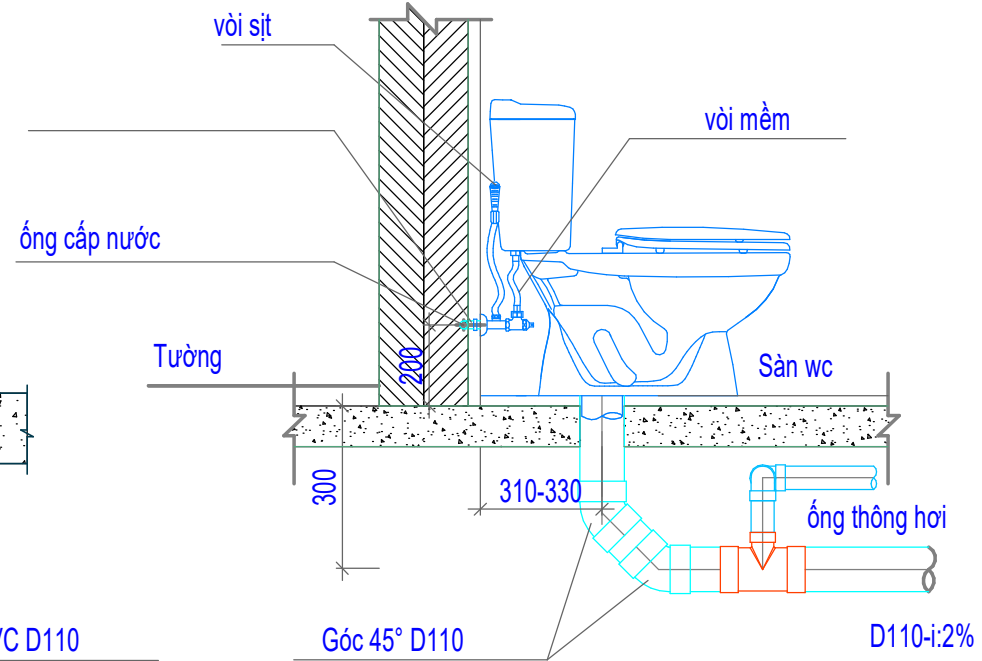
CHI TIẾT LẮP ĐẶT XÍ BỆT TL: ( 1 : 50 )
