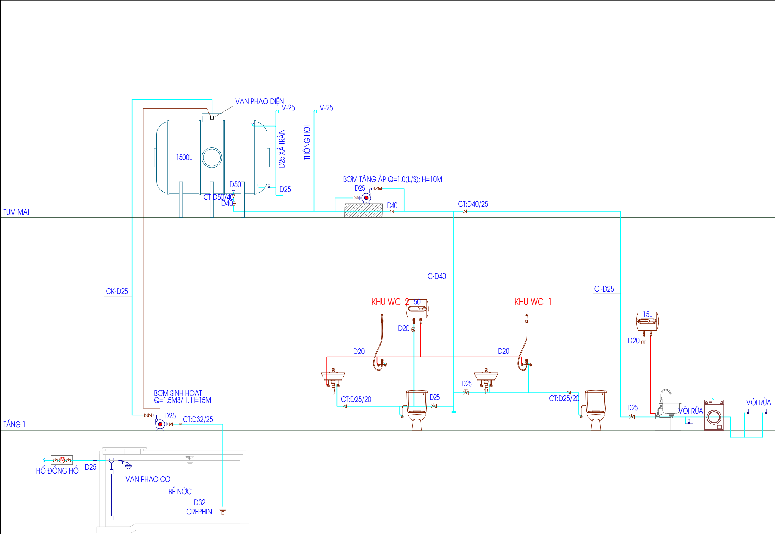
SƠ ĐỒ NGUYÊN LÝ CẤP NƯỚC
