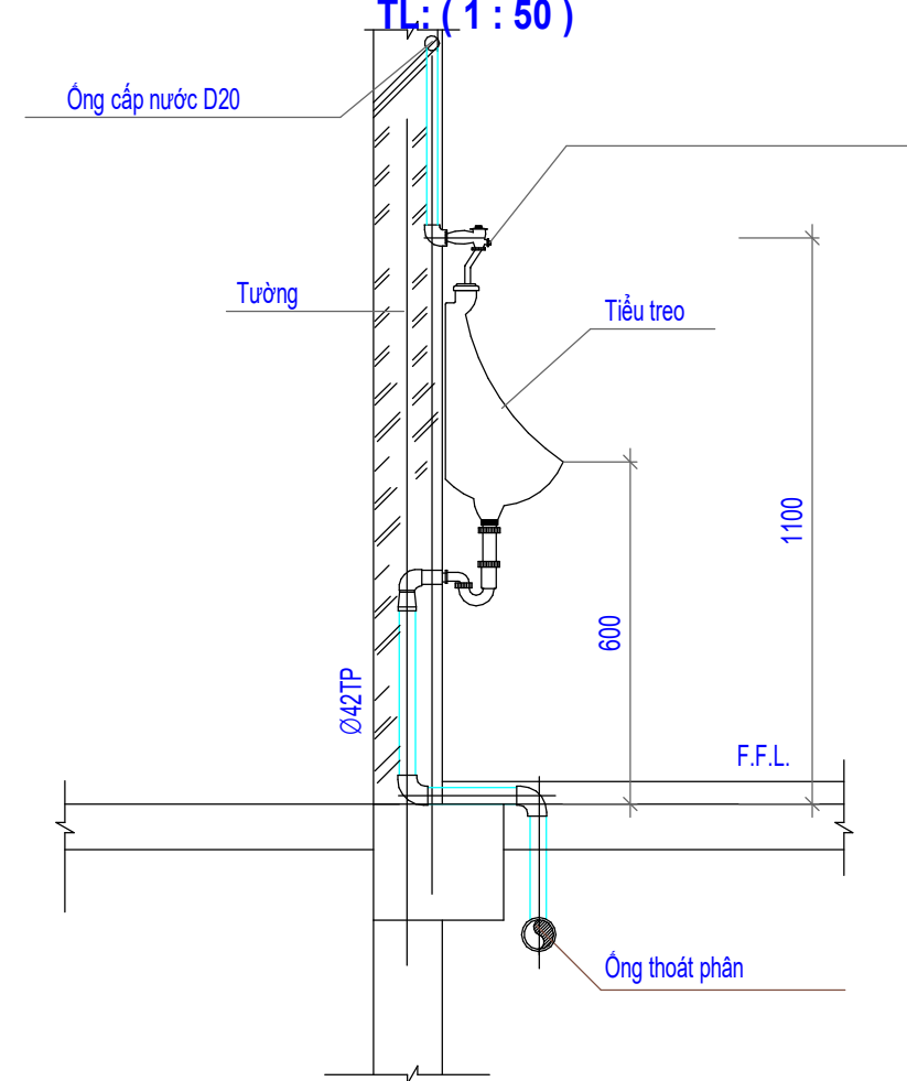
CHI TIẾT LẮP ĐẶT TIỂU NAM TL: ( 1 : 50 )
