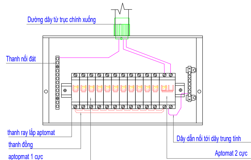
CHI TIẾT APTOMAT CÁC TẦNG
