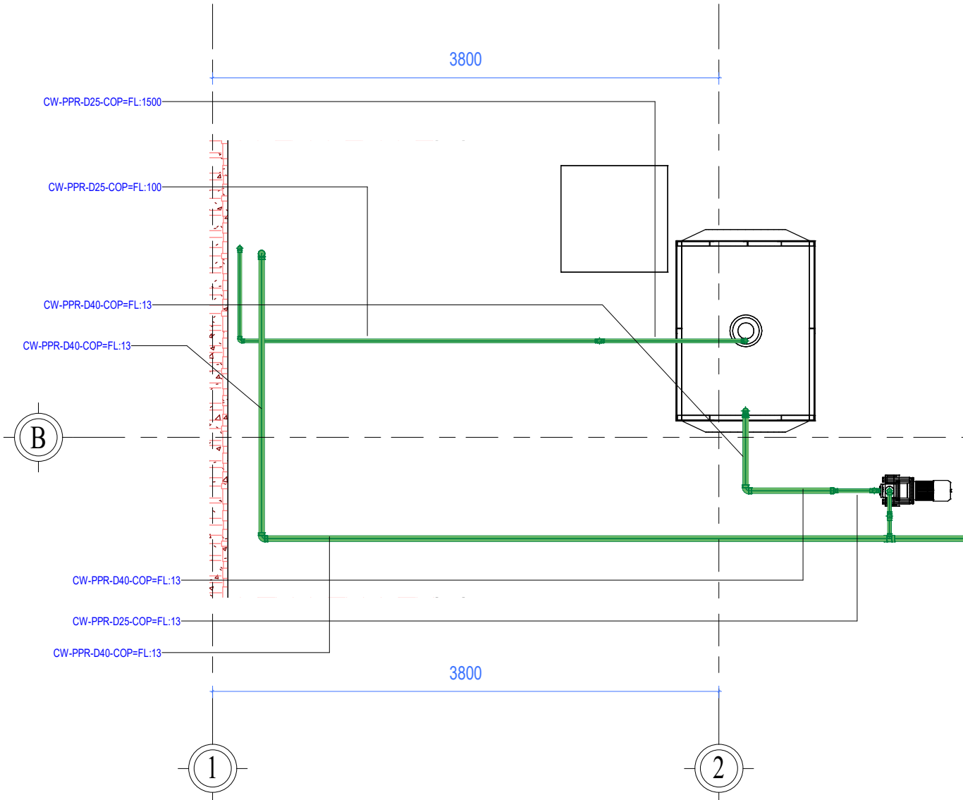
CHI TIẾT CẤP NƯỚC LÊN TẾC TL: ( 1 : 40 )
