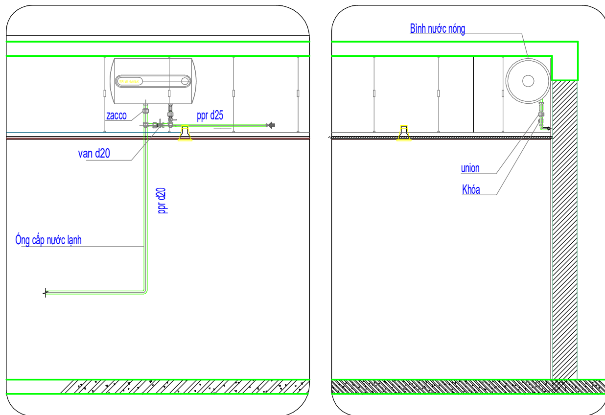
CHI TIẾT LẮP ĐẶT BÌNH NÓNG LẠNH TL: ( 1 : 50 )
