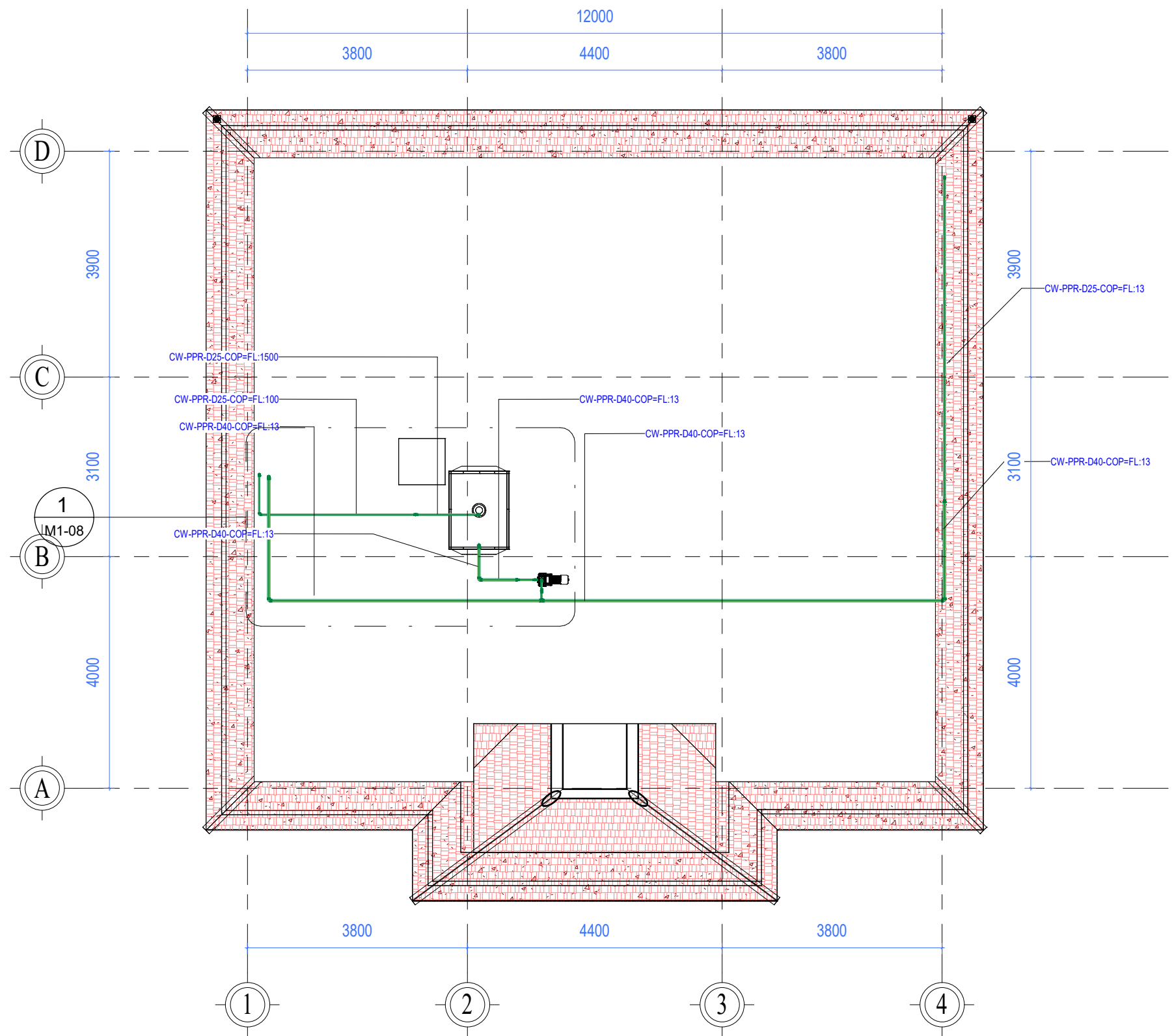
MẶT BẰNG CẤP NƯỚC TẦNG ÁP MÁI TL: (1 : 85)
