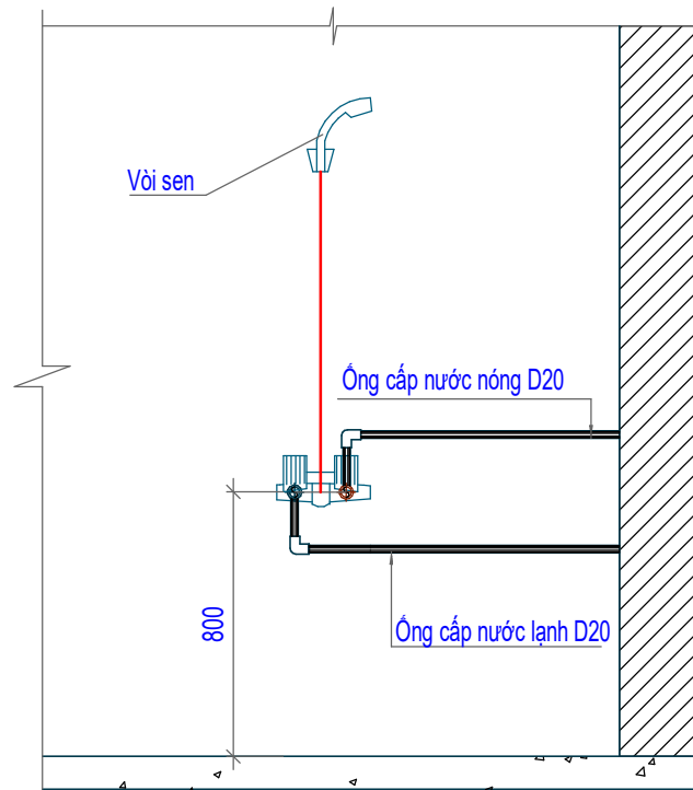
CHI TIẾT LẮP ĐẶT VÒI TẮM TL: ( 1 : 50 )
