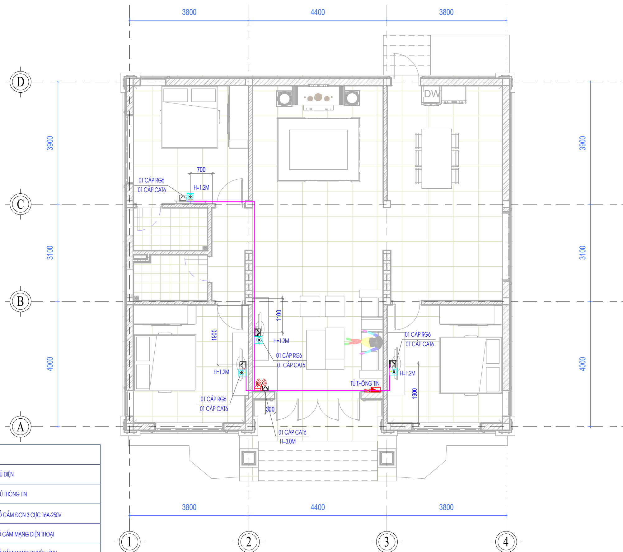
MẶT BẰNG HỆ THỐNG THÔNG TIN TẦNG 1 TL: (1 : 75 )
