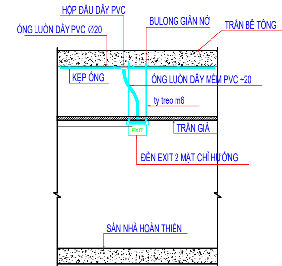
CHI TIẾT ĐÈN EXIT 2 MẶT CHỈ HƯỚNG
