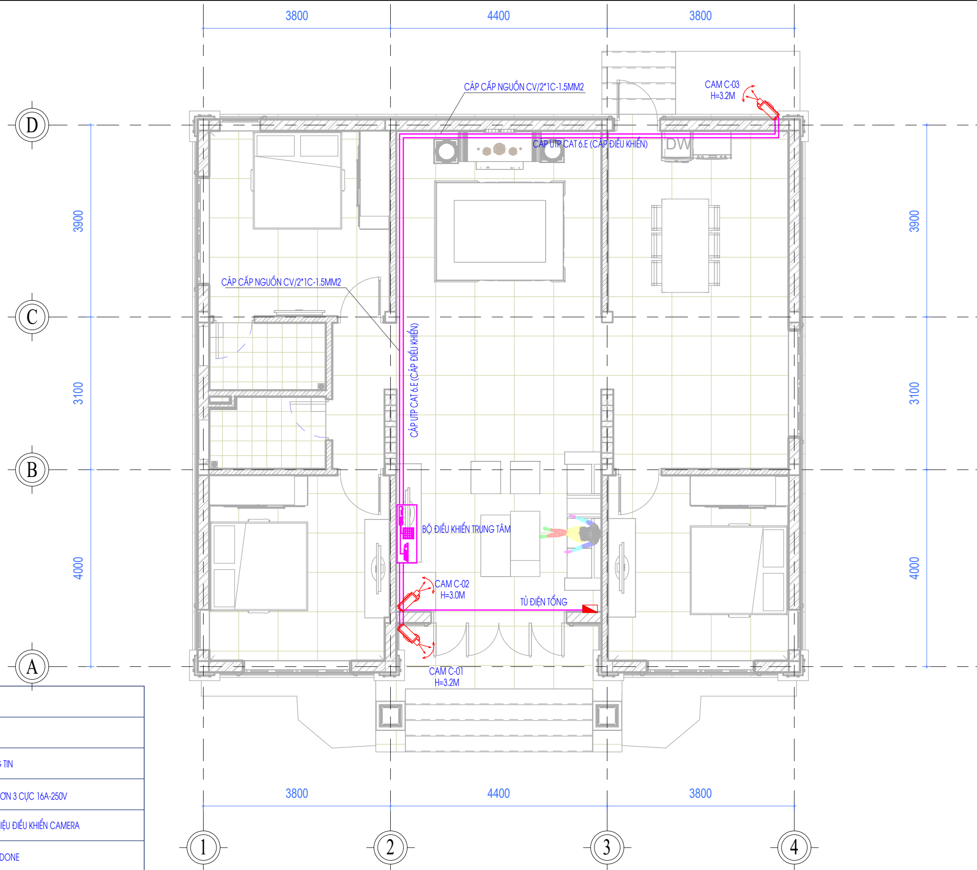
MẶT BẰNG CAMERA TẦNG 1 TL: (1 : 75 )
