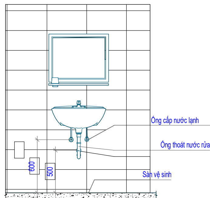
CHI TIẾT LẮP ĐẶT CHẬU RỬA TL: ( 1 : 50 )
