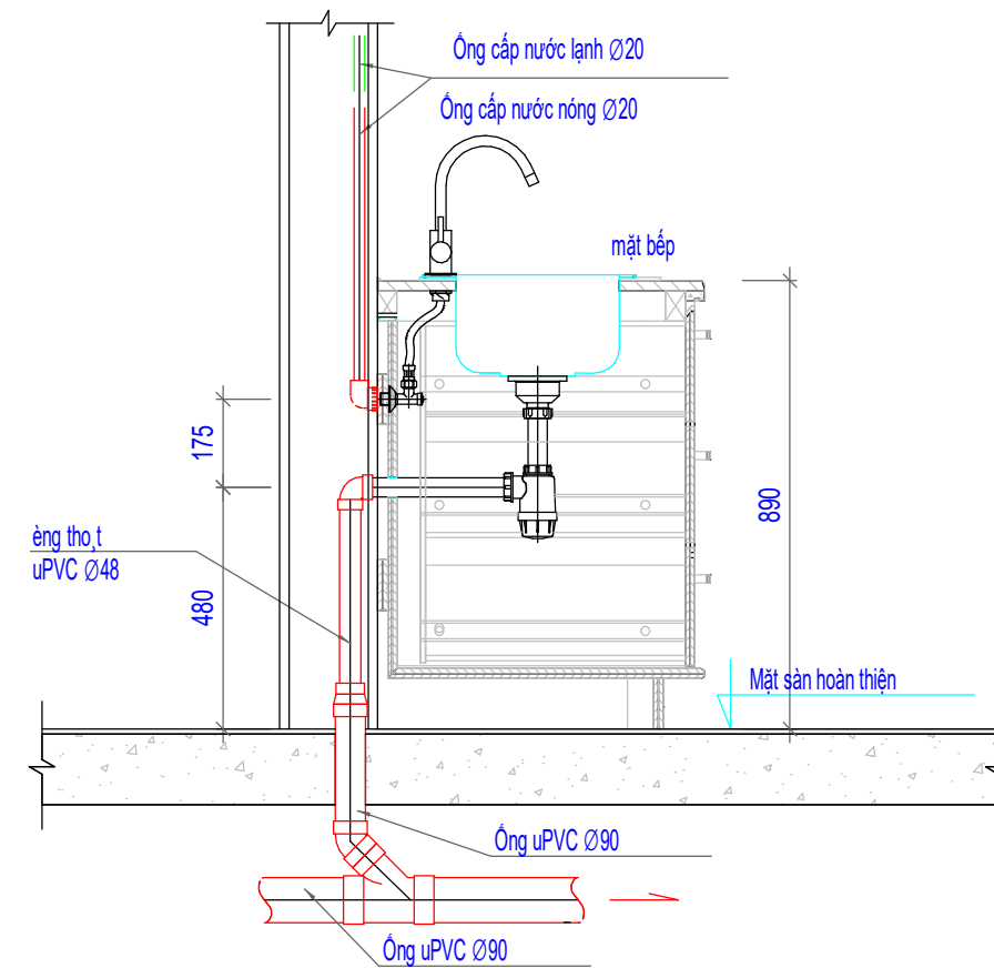
CHI TIẾT LẮP ĐẶT BỒN RỬA BÁT TL: ( 1 : 50 )
