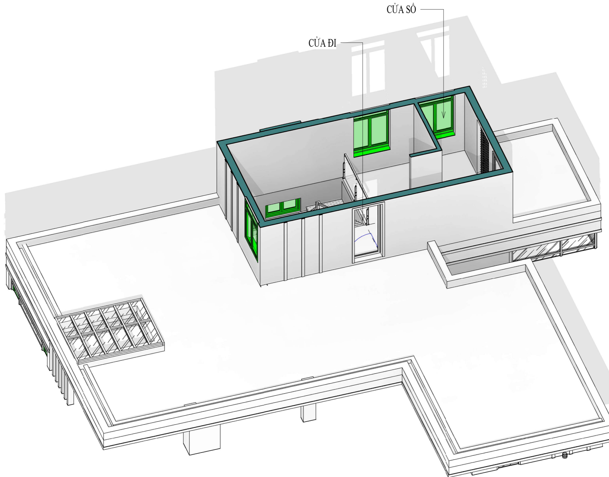
3D MẶT BẰNG BỐ TRÍ CỬA TẦNG 3 TỈ LỆ: ( )
