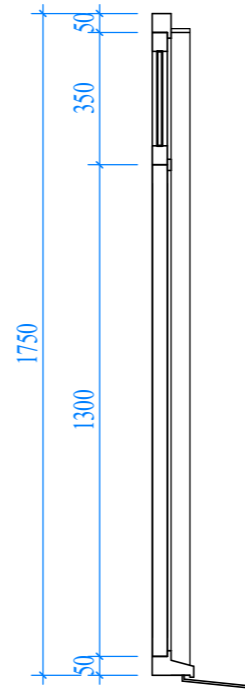
MẶT CẮT TỈ LỆ: ( 1 : 20 )
