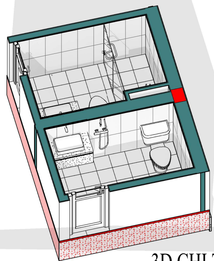
CHI TIẾT WC2,3 TỈ LỆ: (1 : 40)
