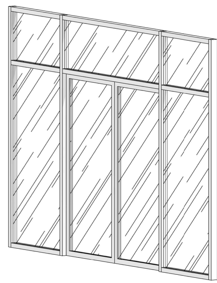
3D CỬA VK11 TỈ LỆ: ( )
