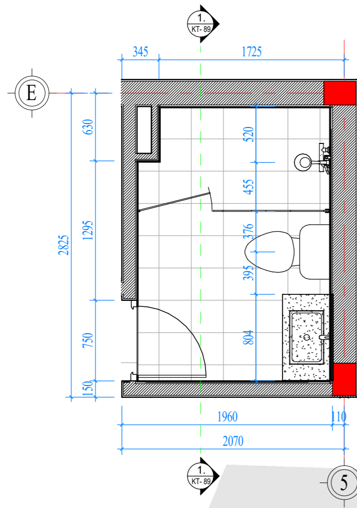
CHI TIẾT WC5 TỈ LỆ: (1 : 35)
