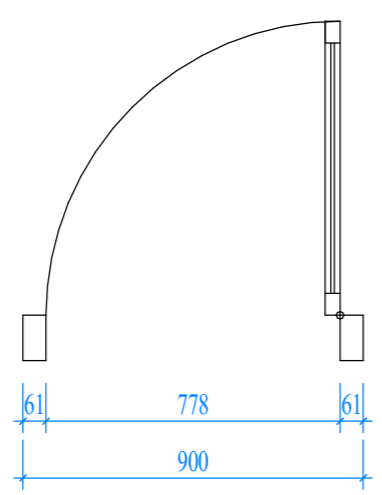
MẶT ĐỨNG TỈ LỆ: ( 1 : 20 )
