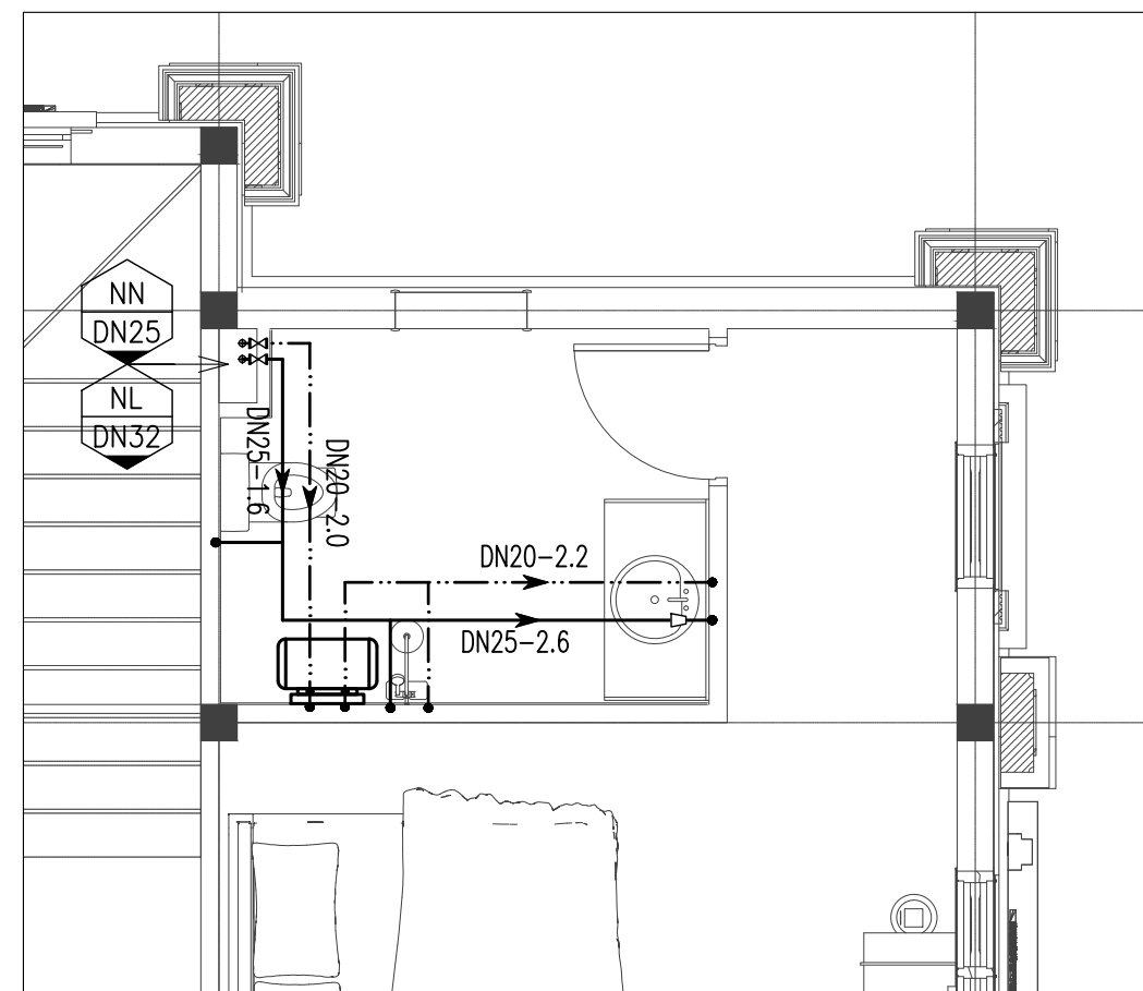
MẶT BẰNG CẤP NƯỚC KHU VỆ SINH - WC03
