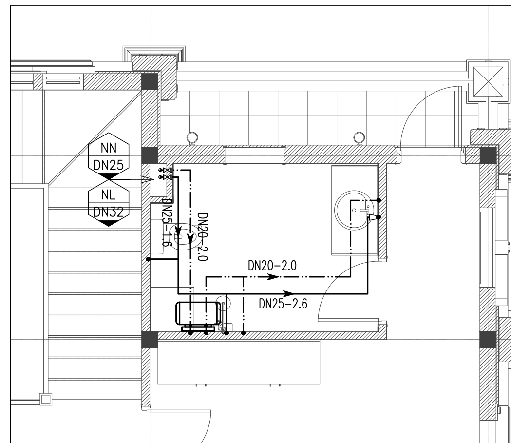
MẶT BẰNG CẤP NƯỚC KHU VỆ SINH - WC07
