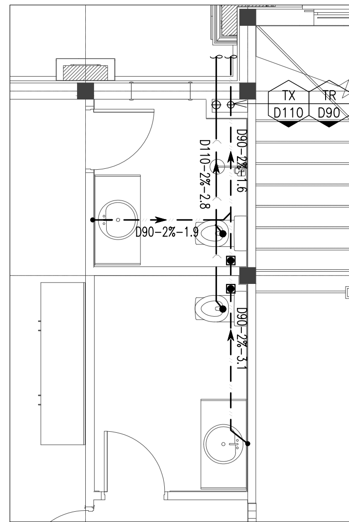
MẶT BẰNG THOÁT NƯỚC KHU VỆ SINH - WC02 TL: 1/50
