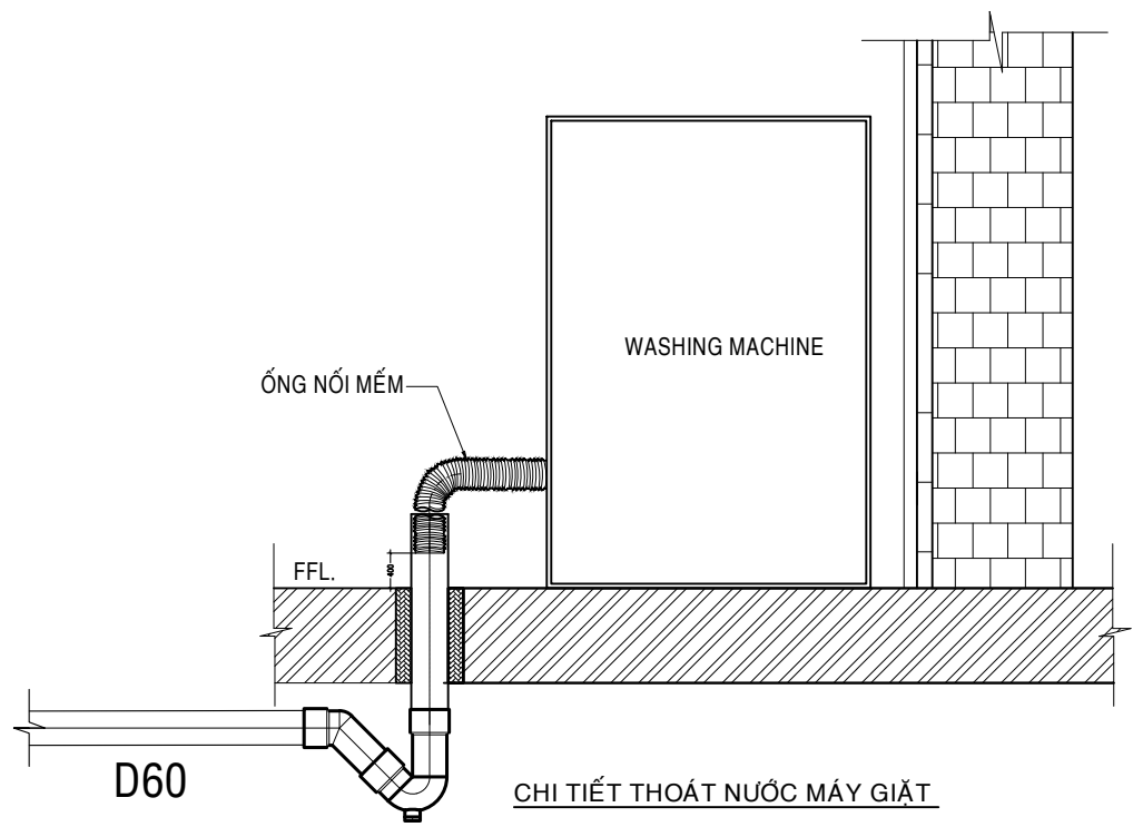
CHI TIẾT LẮP ĐẶT MÁY GIẶT
