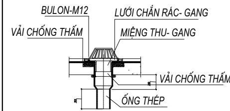
CẦU THU MƯA MÁI
