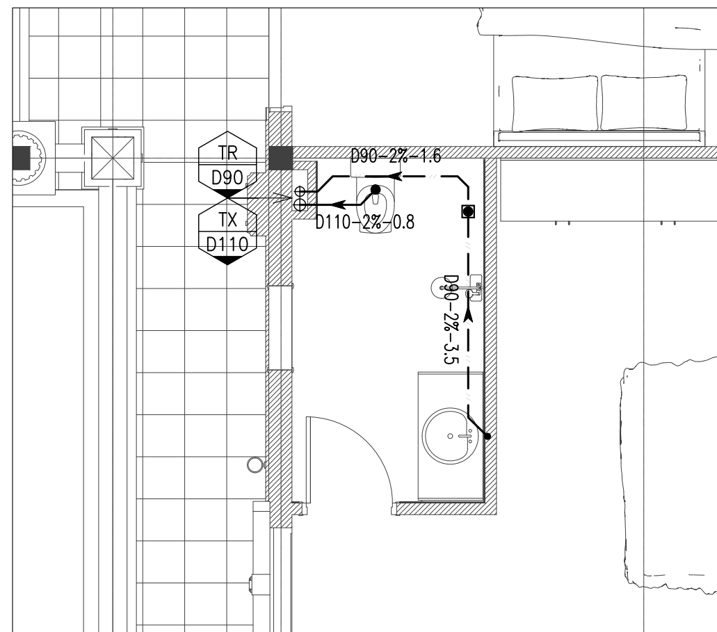
MẶT BẰNG THOÁT NƯỚC KHU VỆ SINH - WC08
