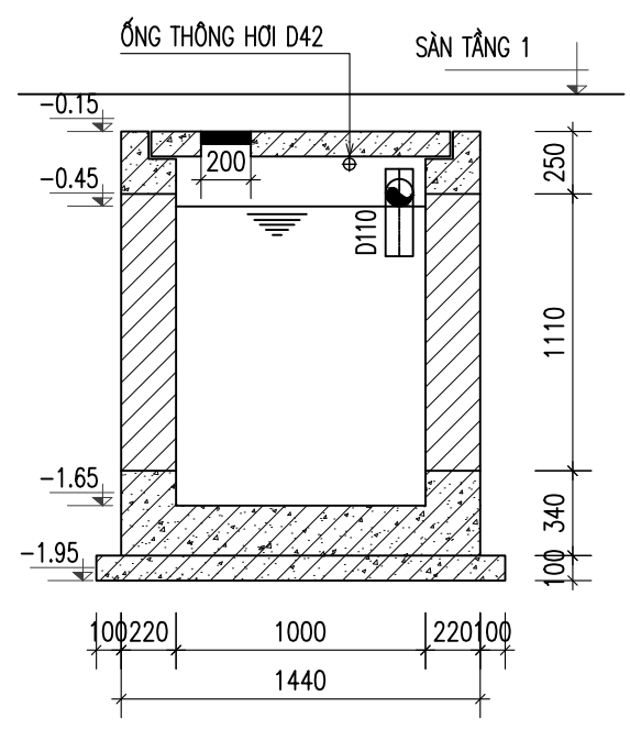
MẶT CẮT 1-1
