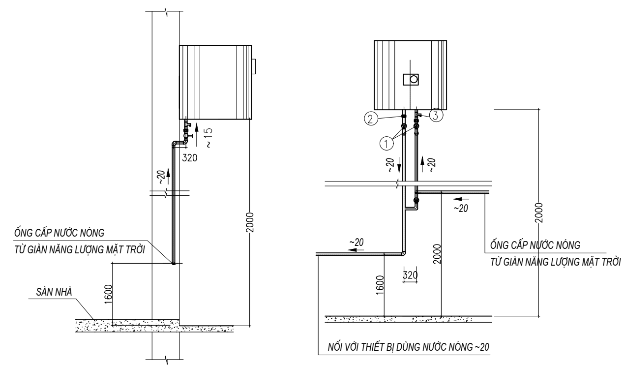
CHI TIẾT LẮP ĐẶT BÌNH NÓNG LẠNH
