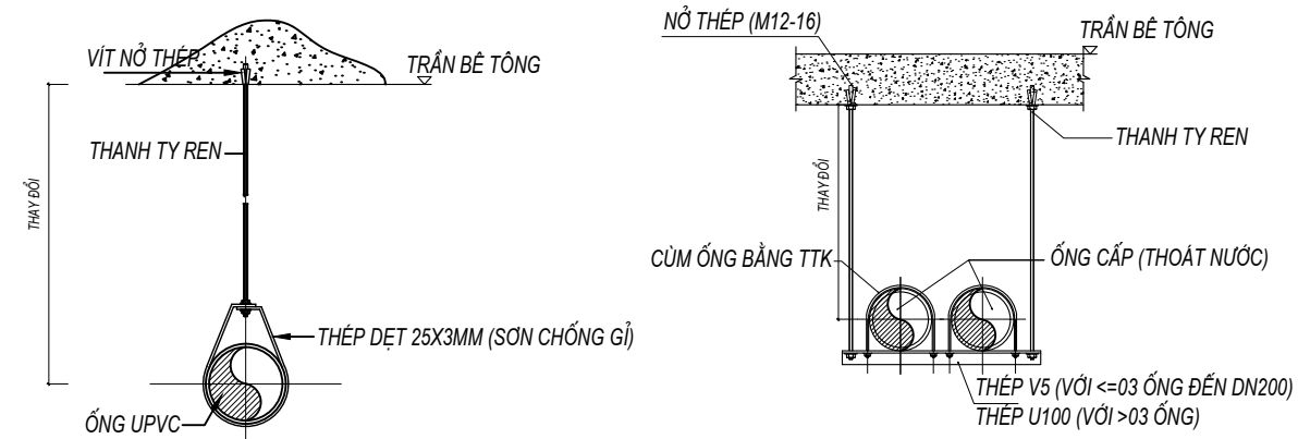
CHI TIẾT CÙM TREO ỚNG THOÁT NƯỚC U.PVC
