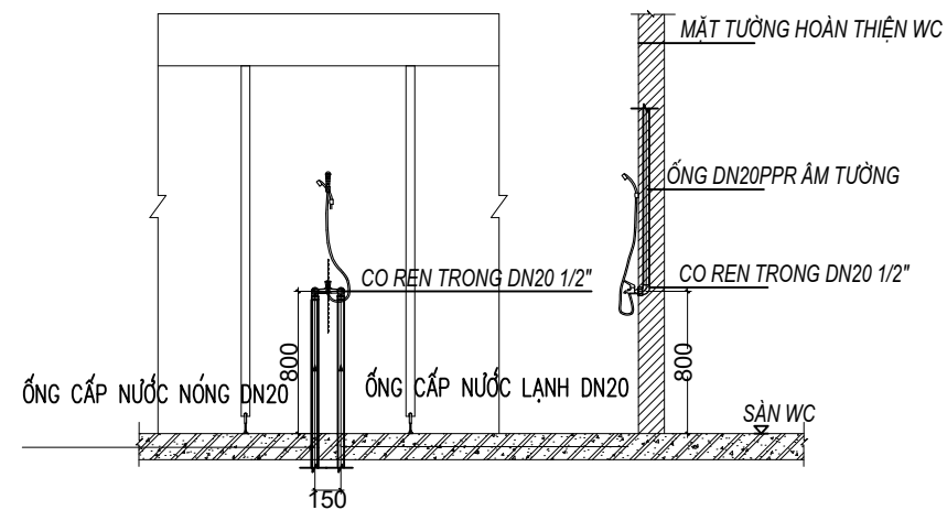
CHI TIẾT LẮP ĐẶT VÒI SEN TẮM ĐỪNG ĐIỂN HÌNH
