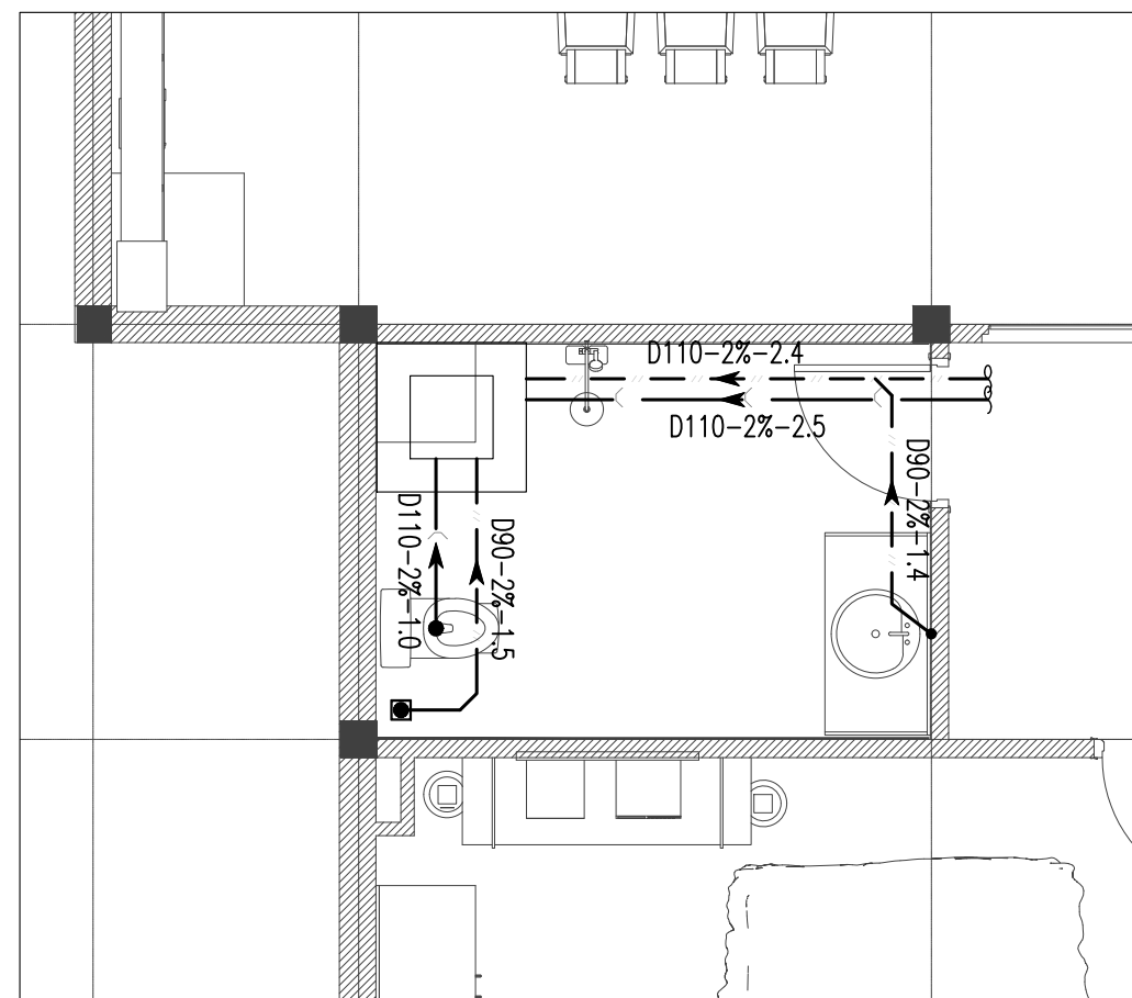
MẶT BẰNG THOÁT NƯỚC KHU VỆ SINH - WC01
