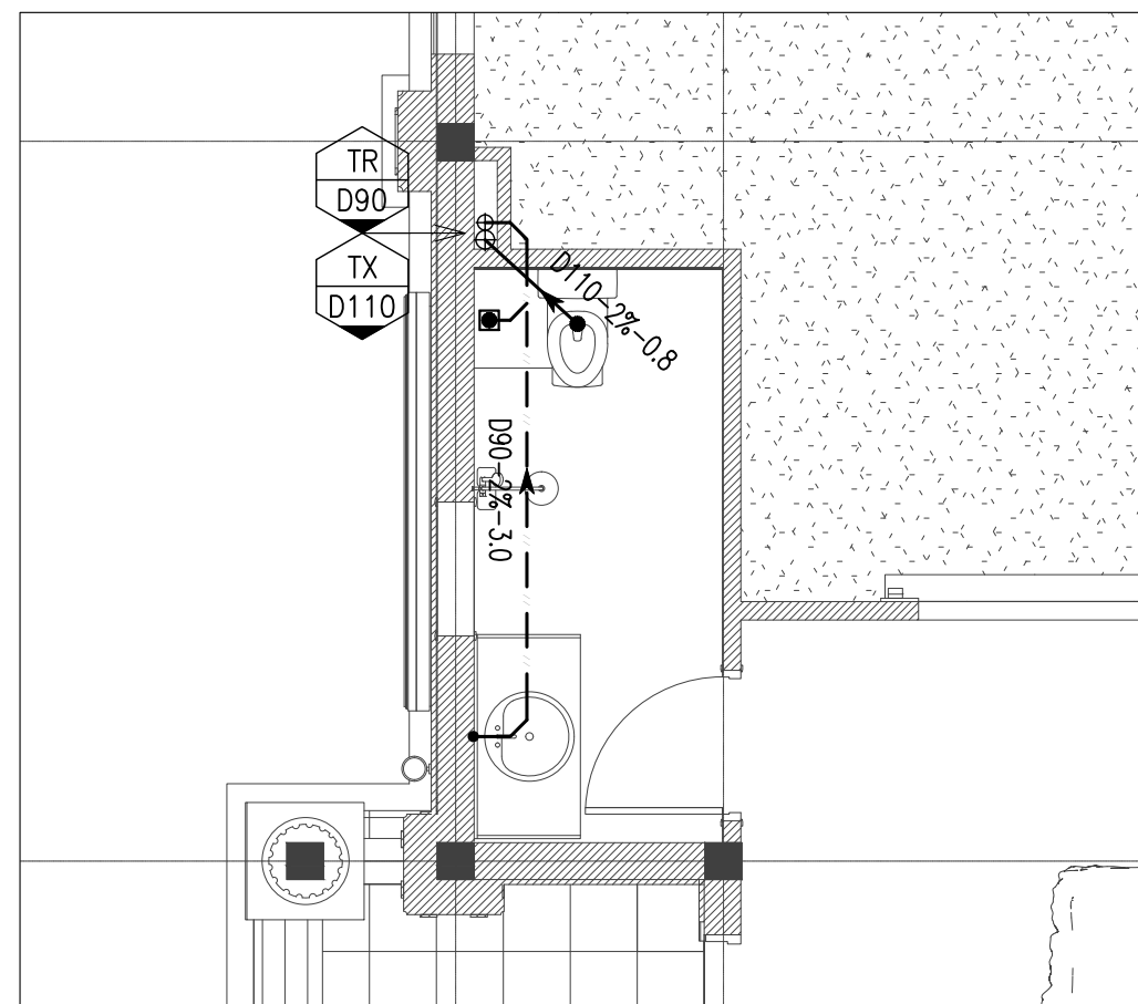
MẶT BẰNG THOÁT NƯỚC KHU VỆ SINH - WC05
