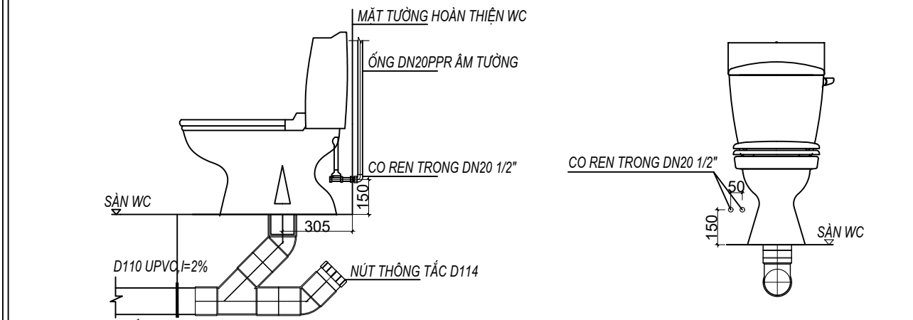
CHI TIẾT LẮP ĐẶT THIẾT BỊ XÍ BỆT ĐIỂN HÌNH
