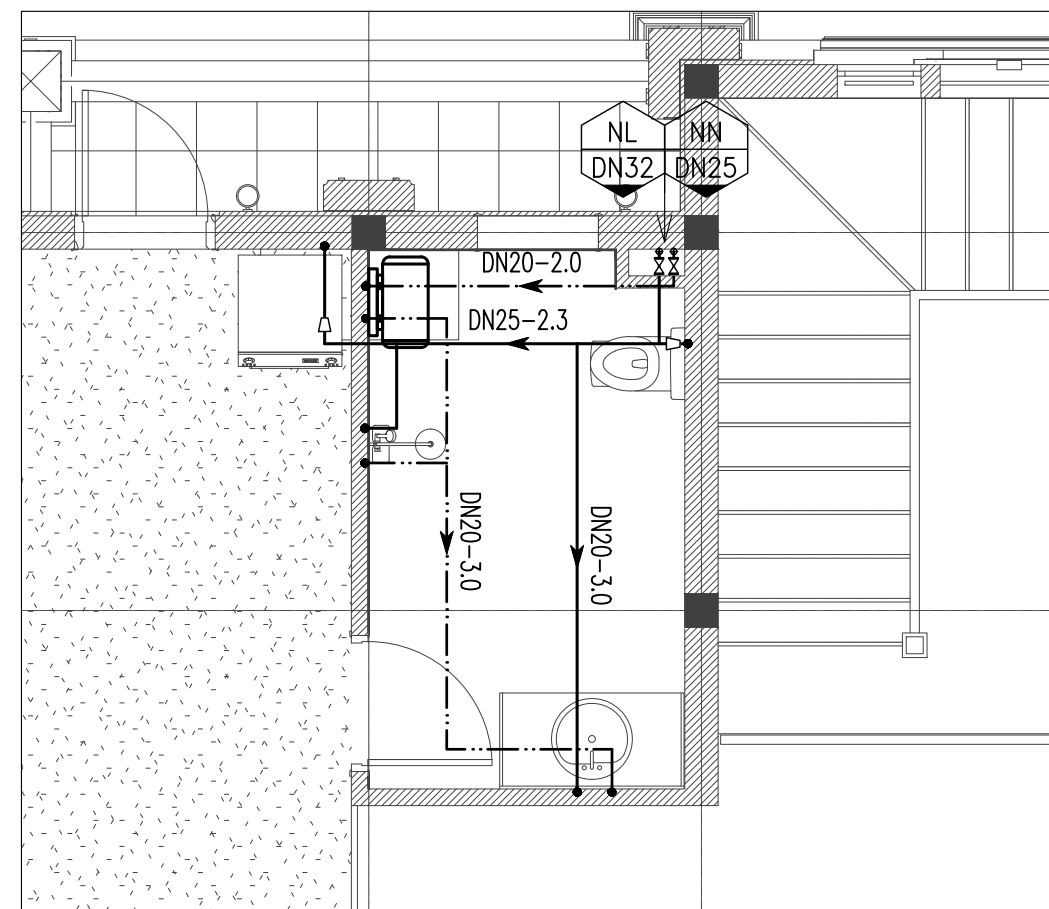
MẶT BẰNG CẤP NƯỚC KHU VỆ SINH - WC06
