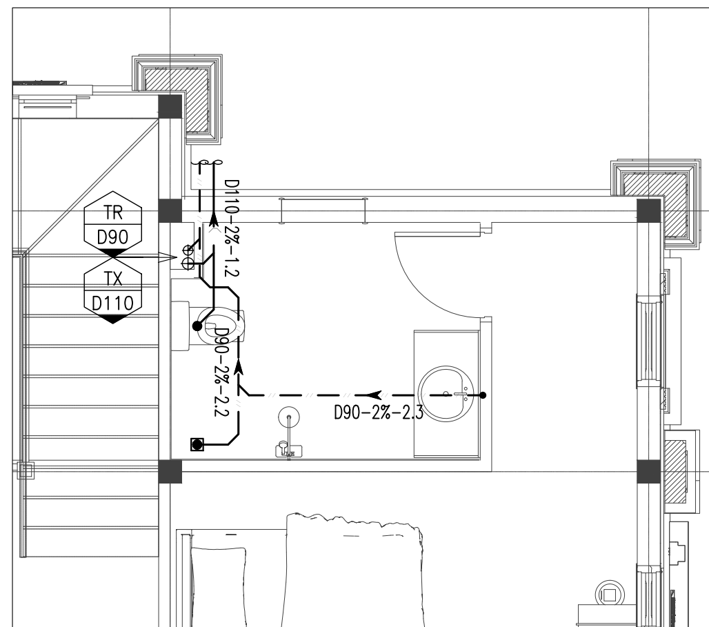
MẶT BẰNG THOÁT NƯỚC KHU VỆ SINH - WC03
