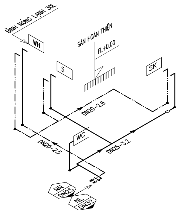
SƠ ĐỒ KHÔNG GIAN CẤP NƯỚC KHU VỆ SINH - WC01
