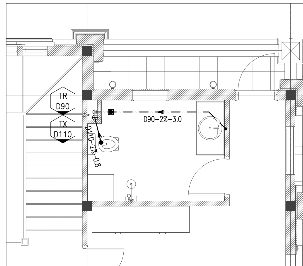
MẶT BẰNG THOÁT NƯỚC KHU VỆ SINH - WC07
