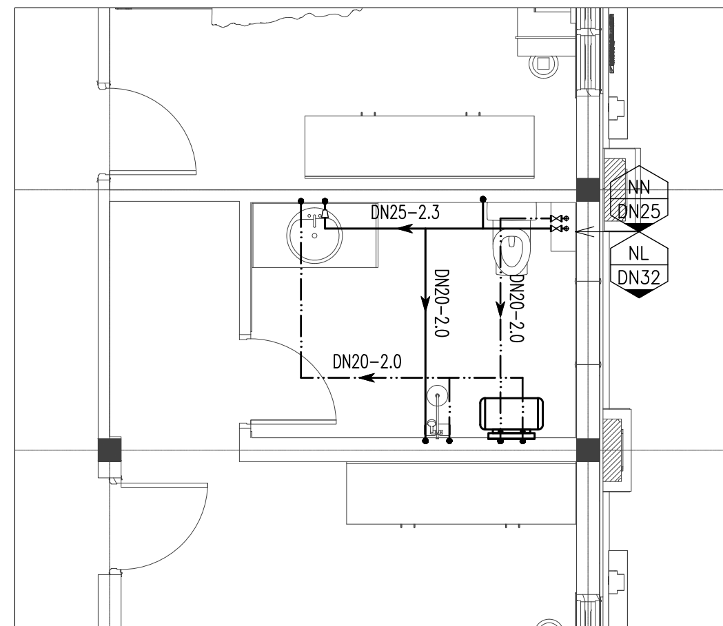
MẶT BẰNG CẤP NƯỚC KHU VỆ SINH - WC04
