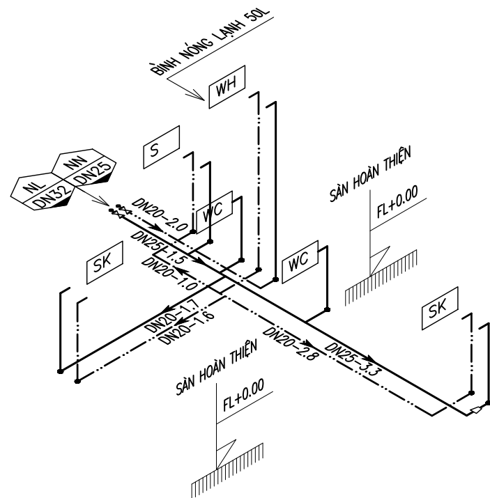
SƠ ĐỒ KHÔNG GIAN CẤP NƯỚC KHU VỆ SINH - WC02
