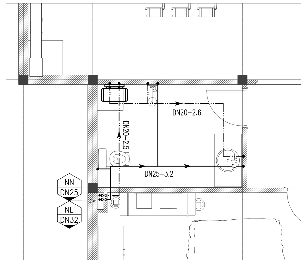
MẶT BẰNG CẤP NƯỚC KHU VỆ SINH - WC01
