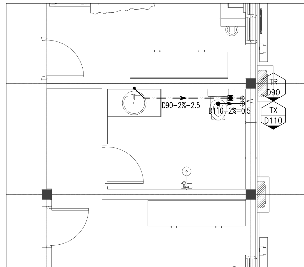
MẶT BẰNG THOÁT NƯỚC KHU VỆ SINH - WC04
