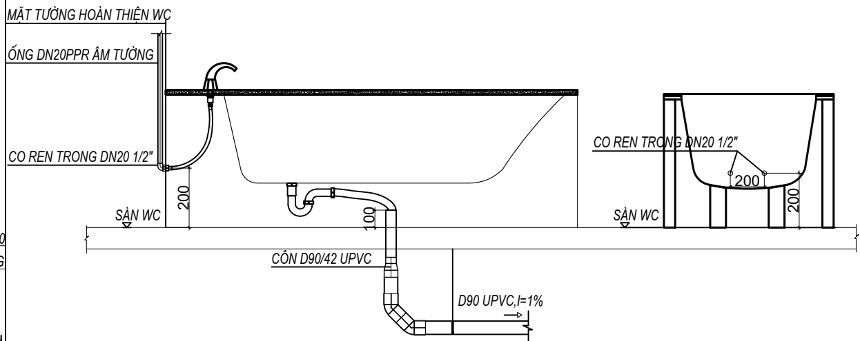
CHI TIẾT LẮP ĐẶT THIẾT BỊ BỒN TẮM ĐIỂN HÌNH
