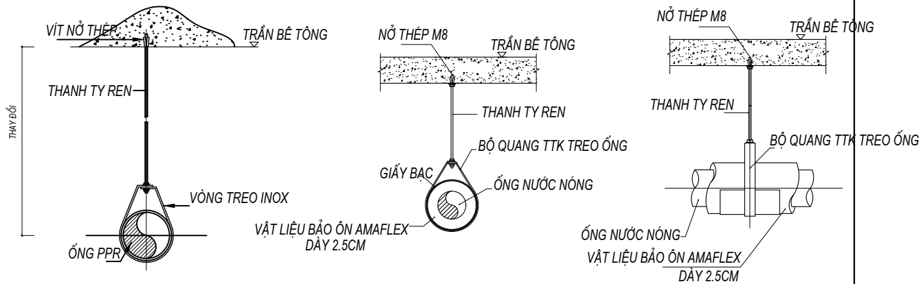
CHI TIẾT CÙM TREO ỚNG NƯỚC PPR
