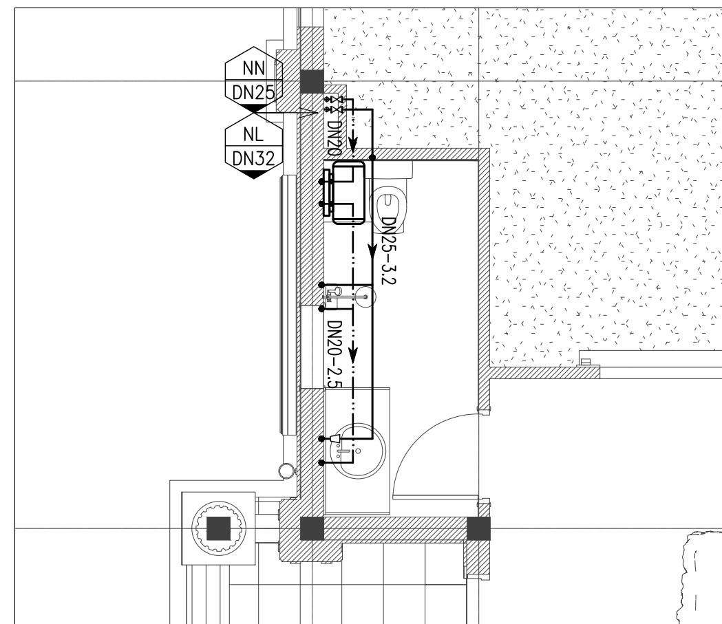
MẶT BẰNG CẤP NƯỚC KHU VỆ SINH - WC05
