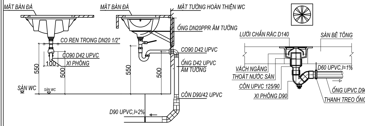
CHI TIẾT LẮP ĐẶT LAVABO ÂM BÀN ĐÁ ĐIỂN HÌNH
