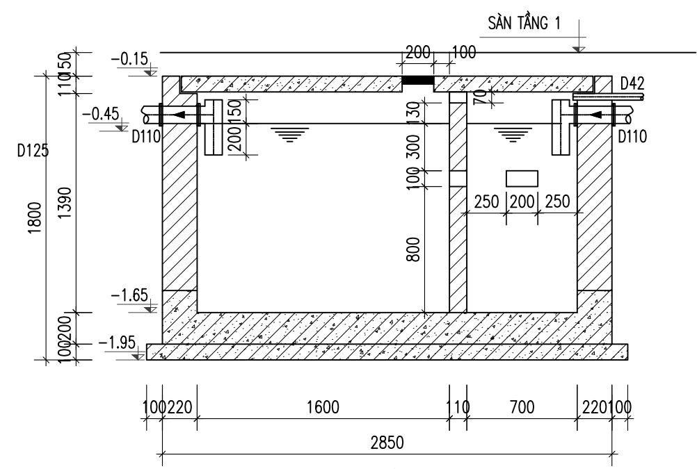
MẶT CẮT 2-2
