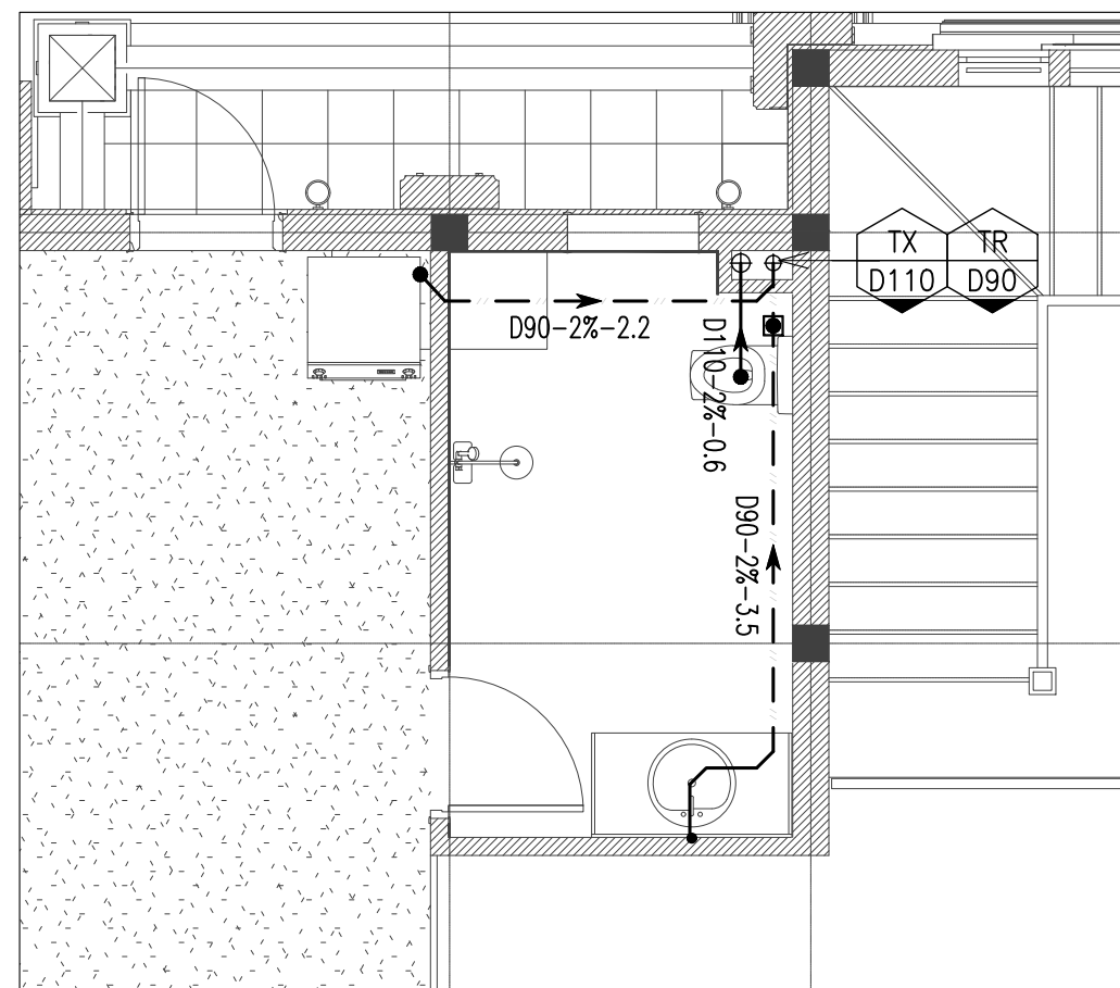
MẶT BẰNG THOÁT NƯỚC KHU VỆ SINH - WC06
