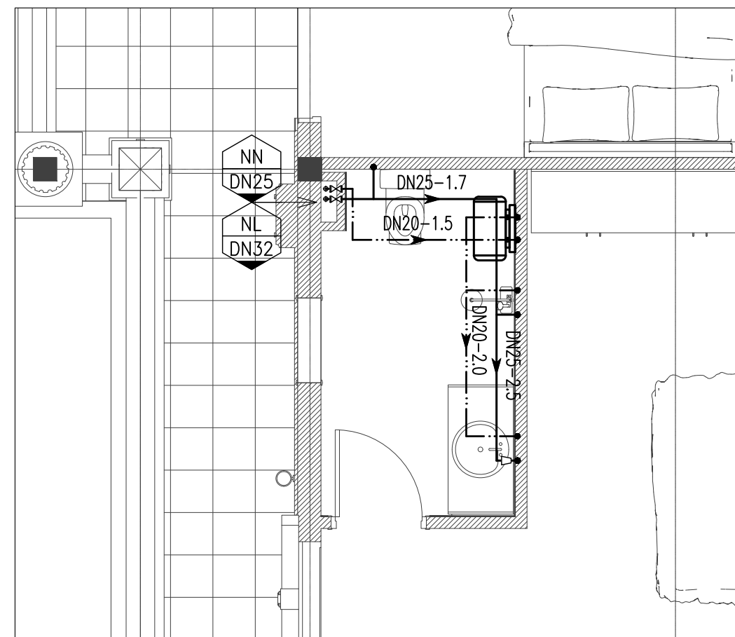
MẶT BẰNG CẤP NƯỚC KHU VỆ SINH - WC08
