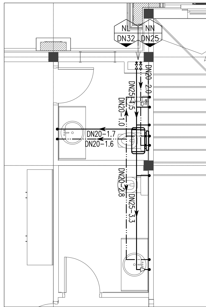
MẶT BẰNG CẤP NƯỚC KHU VỆ SINH - WC02 TL: 1/50
