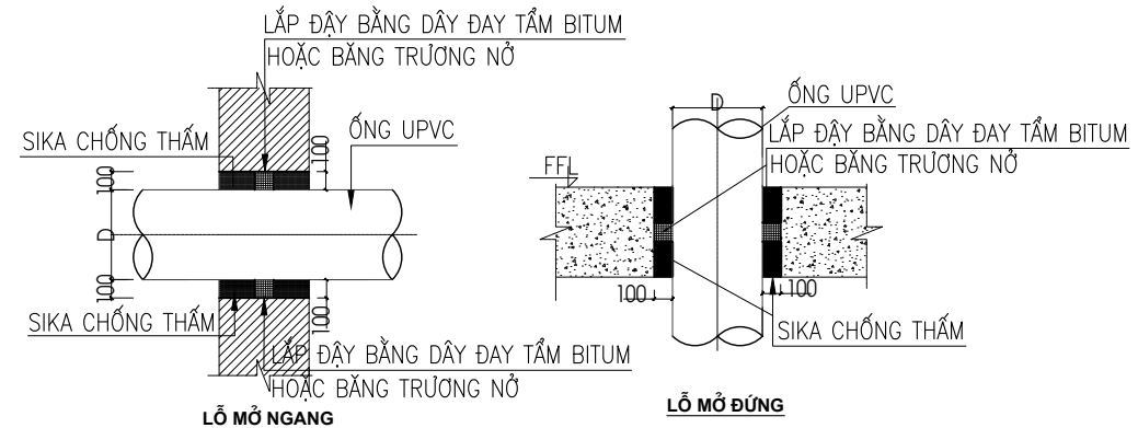
CHI TIẾT ĐIỂN HÌNH ỚNG U.PVC PPR QUA TƯỜNG, SÀN
